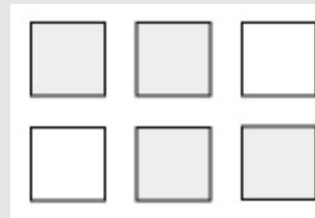
Paare-Spiel
