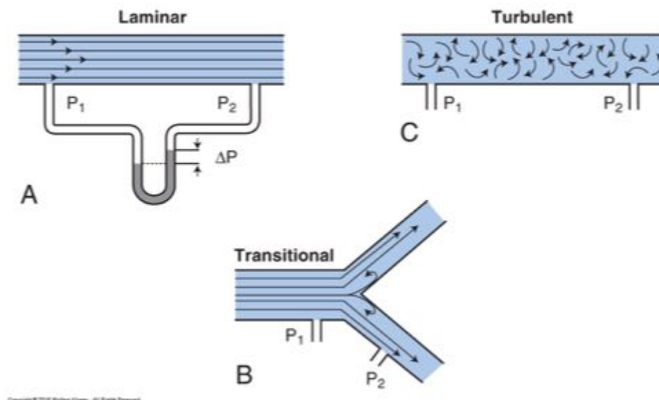
Laminare (A) und turbulente (C) Strömung, sowie Strömung bei Verzweigung der Atemwege (B). Quelle: West & Lucks. Pulmonary Physiology. WolterKluwers Verlag.
