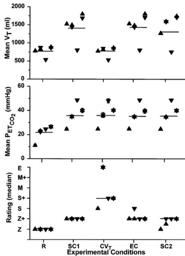
Atemnot-Rating bei 24-h-beatmeten Tetraplegikern in Abhängigkeit der Atemtiefe bei konstant erhöhtem P_{ETCO_2} . R: Ruhe, SC1: 1. Subject Control - Bedingung; CVT: constant tidal volume; EC: Experimentier Control Bedingung; SC2: 2. Subject Control - Bedingung. Quelle: Bloch, Spengler et al. Am J Crit Care Med (1998).
