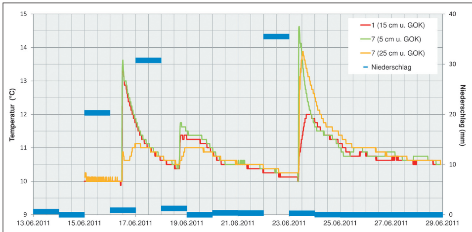
Fig. 7: Gemessener Temperaturverlauf der drei Sensoren (iButtons TM ) in den Rohren 1 (~ 15 cm im Bachsediment) und 7 (~ 5 cm und ~ 25 cm im Bachsediment am Beginn der Messkampagne) sowie der mittlere Niederschlag gemessen an sechs Stationen der Region. Die Temperaturpulse korrelieren deutlich mit den Niederschlagsereignissen.
